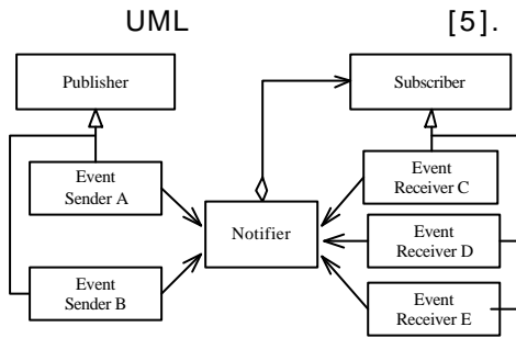
1. UML
